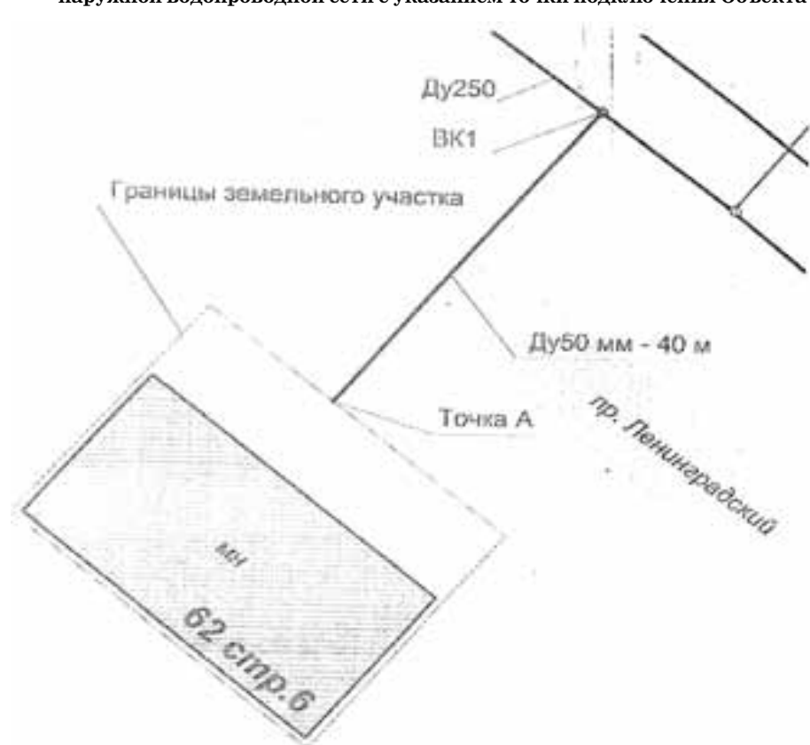
СХЕМА наружной водопроводной сети с указанием точки подключения Объекта
